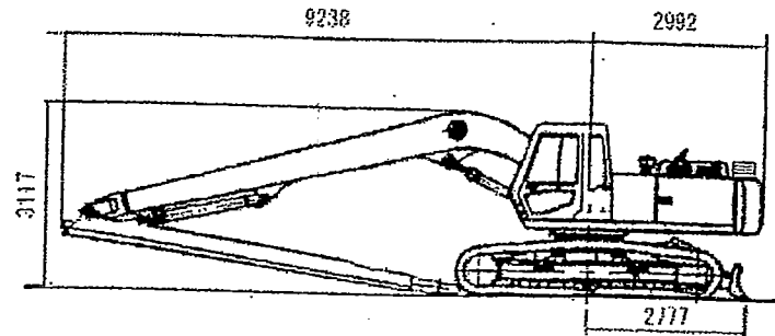
輸送時姿勢
